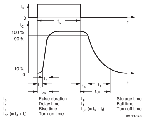
図 4 - 切換時間
