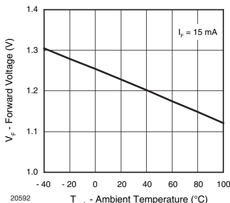
図 6 - 順電圧 VS. 周囲温度
