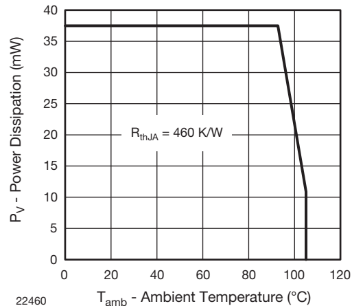
図 1 - 許容損失 VS. 周囲温度
