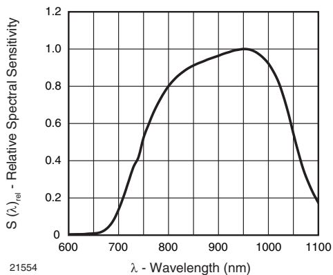
図 5 - 分光感度特性
