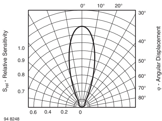
図 6 - 相対放射強度 対 角変位
