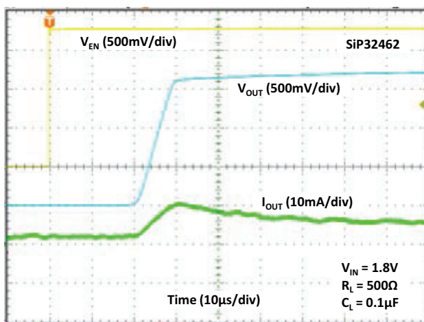
Fig. 28 - Turn-on Time
