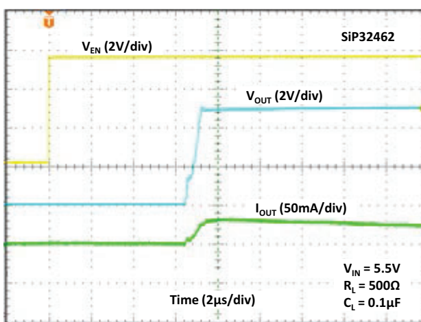
Fig. 31 - Turn-on Time
