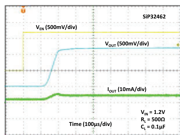
Fig. 30 - Turn-on Time
