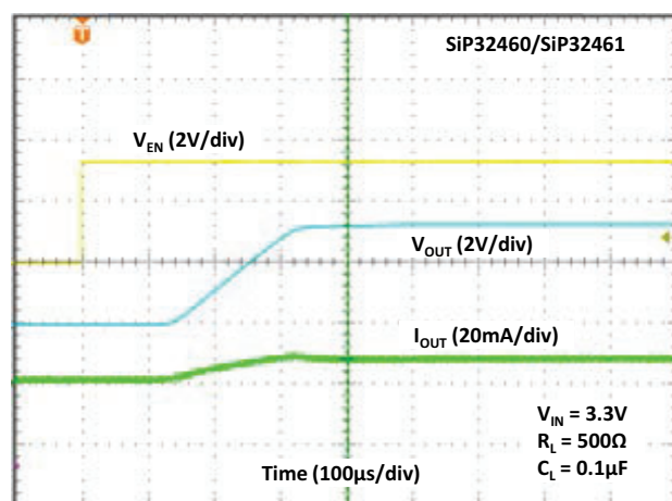
Fig. 27 - Turn-on Time
